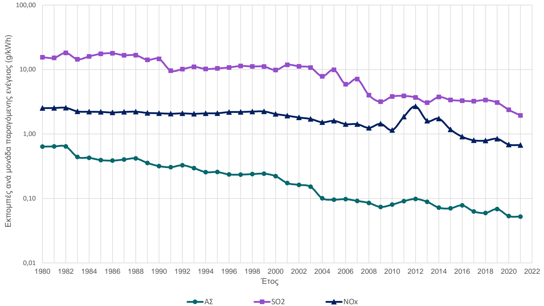
Γράφημα - Ετήσια διακύμανση περιβαλλοντικών δεικτών εκπομπών ΑΣ, SO 2 , NO x σε γραμμάρια ανά κιλοβατώρα από συμβατικές μονάδες ηλεκτροπαραγωγής μεγάλης κλίμακας (λογαριθμική κλίμακα)
